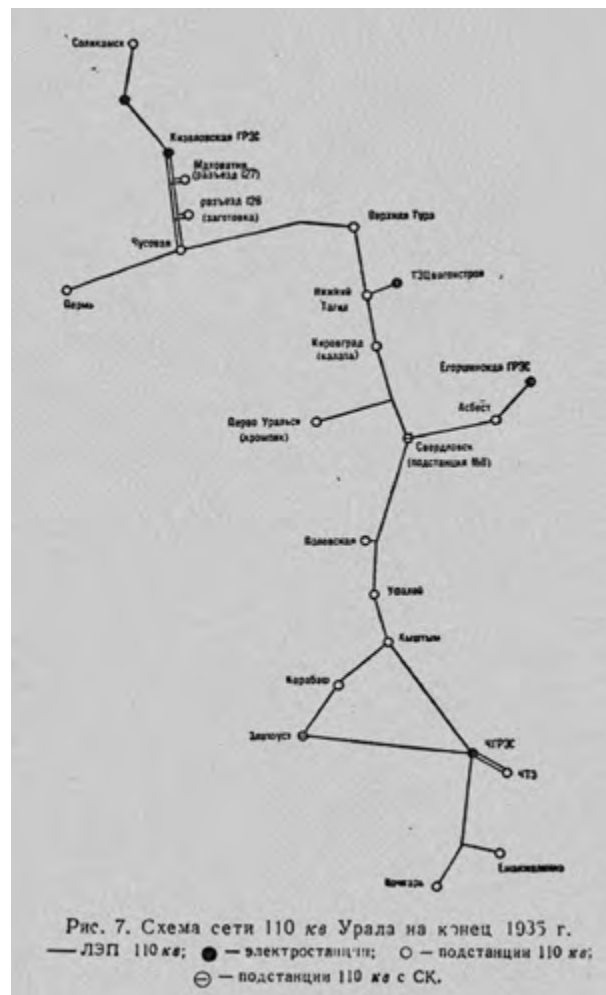
Схема сети 110 кВ Урала на конец 1935 г.
