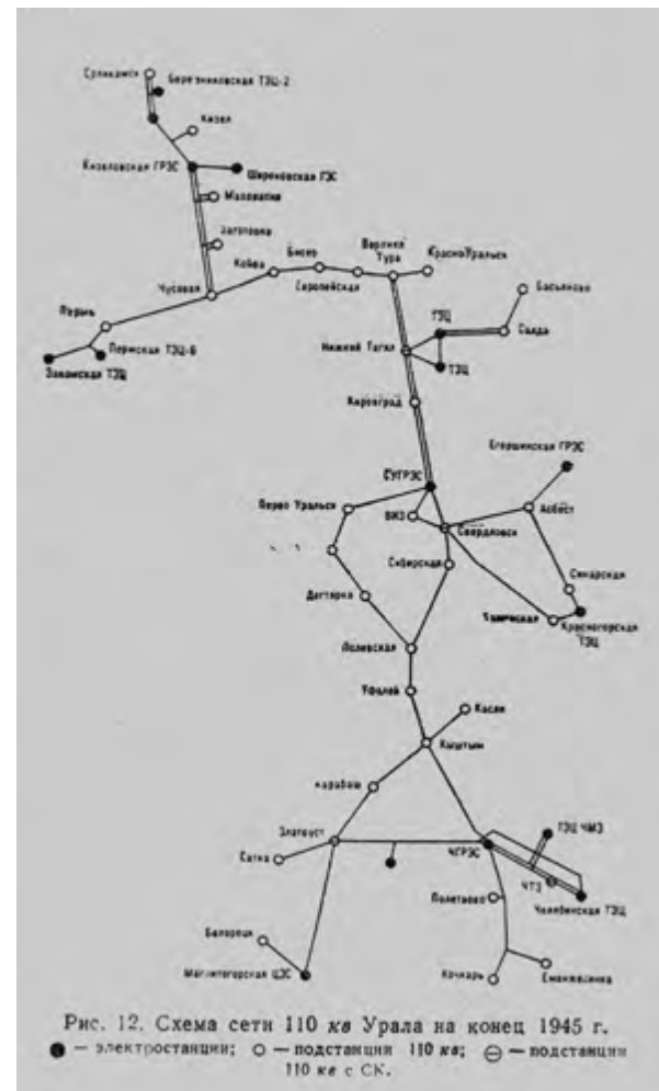
Схема сети 110 кВ Урала на конец 1945 г.
