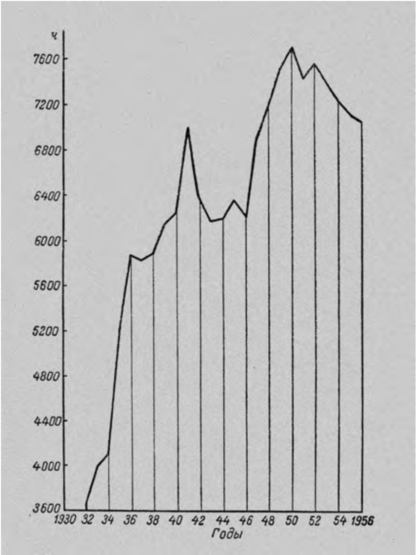
Годовое число часов использования установленной мощности электростанций Уральской энергетической системы (электростанции МЭС)
