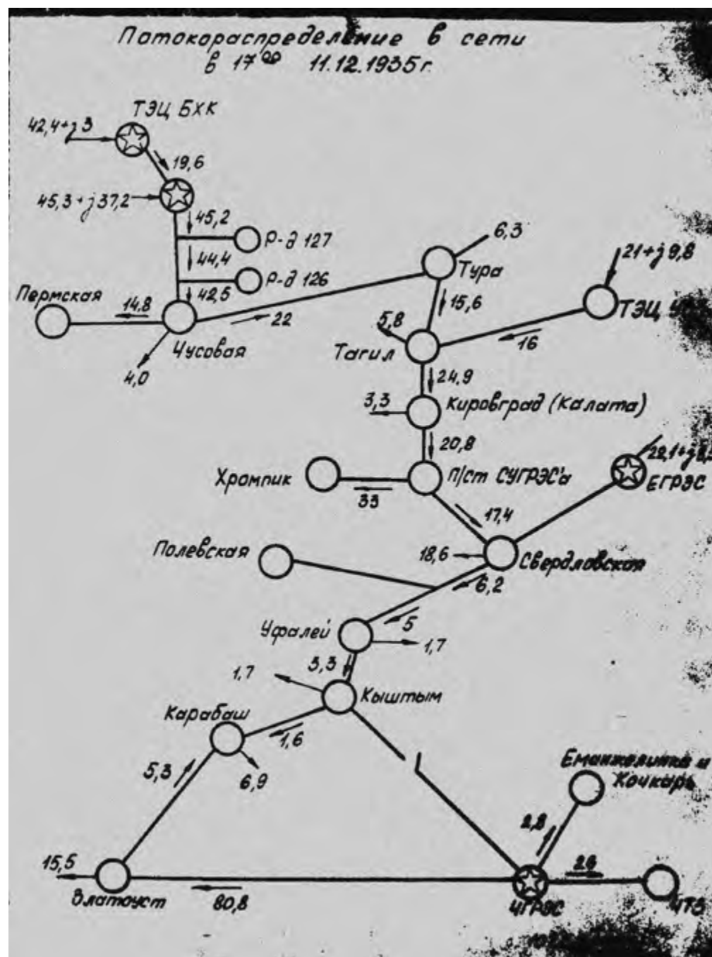
Потокораспределение в сети, 1935 год
